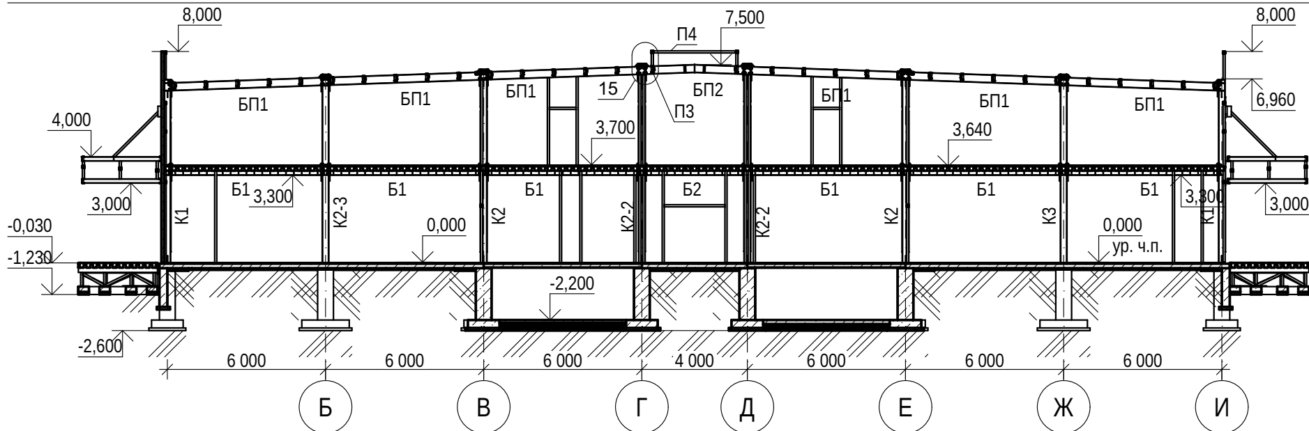
РАЗРЕЗ 4-4
