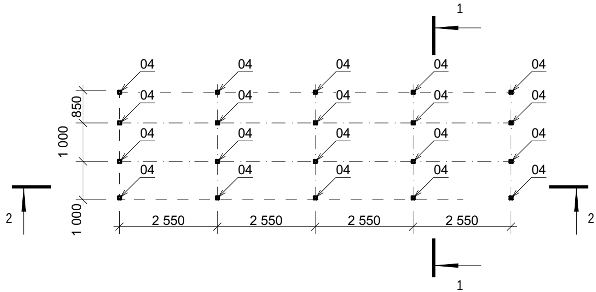
СХЕМА БАЛОК ПЛОЩАДКИ
