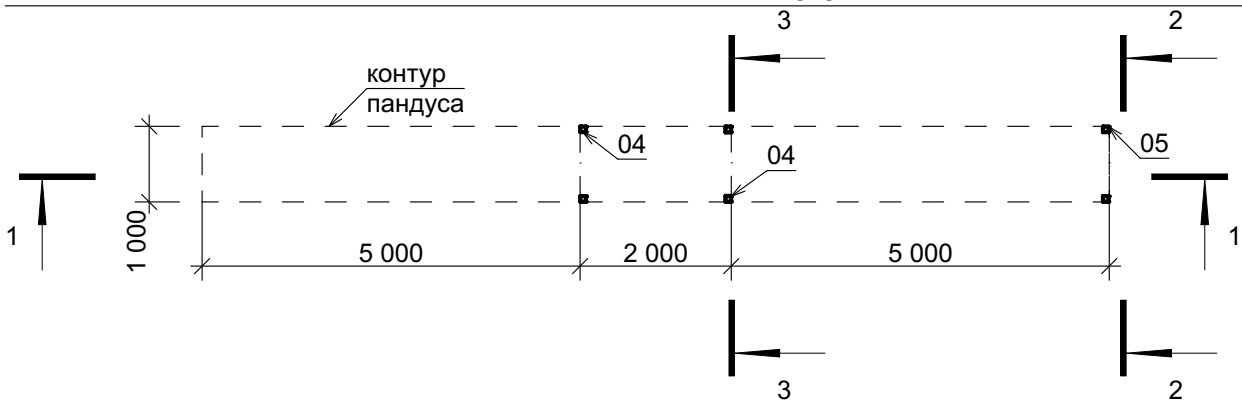
СХЕМА СТОЕК ПАНДУСА 1:100
