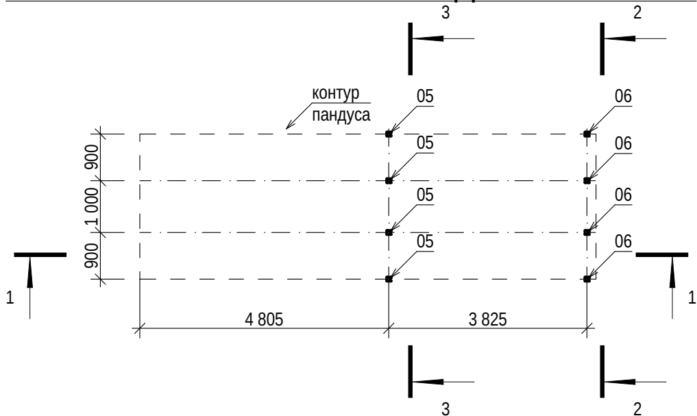
СХЕМА ЛИСТОВ ПОКРЫТИЯ 1:100
