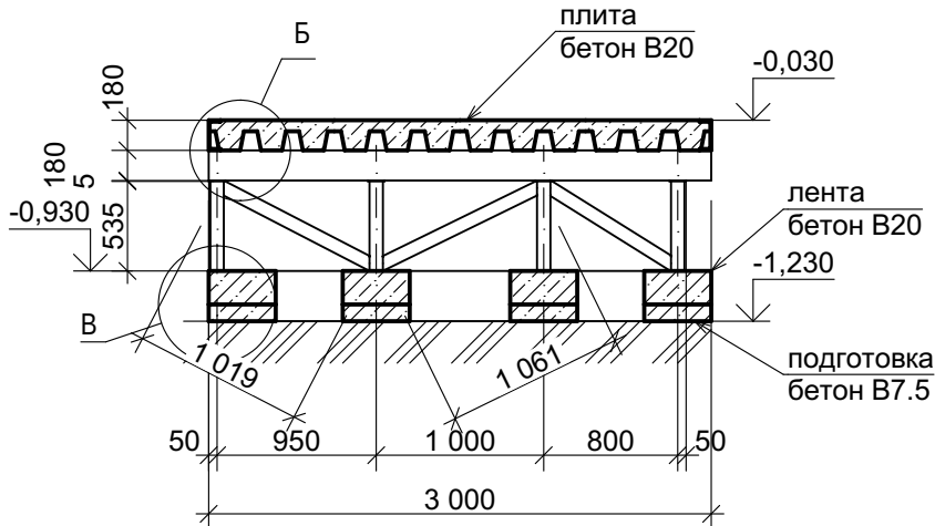
1-1 1:50
