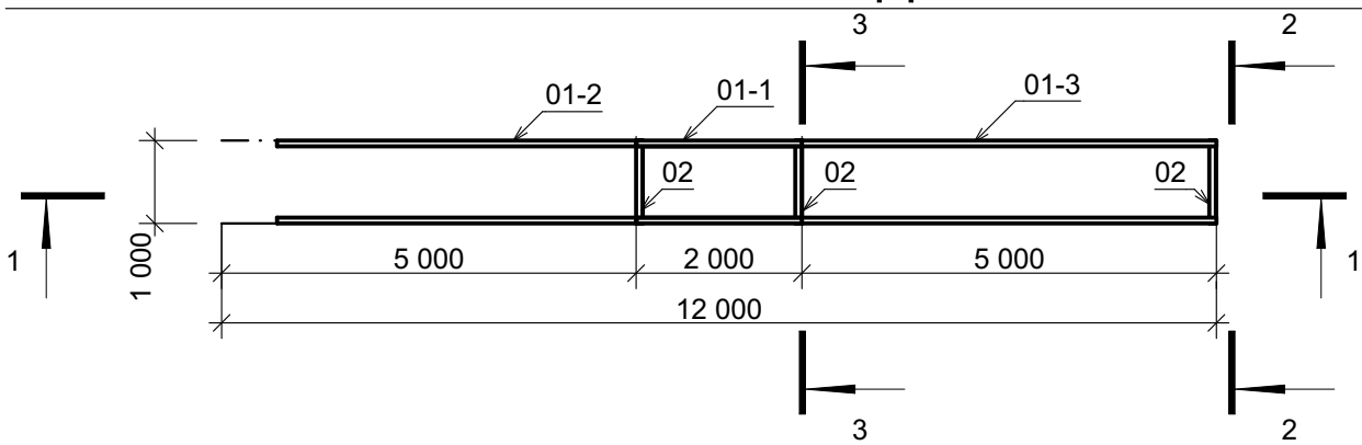
СХЕМА БАЛОК ПАНДУСА 1:100
