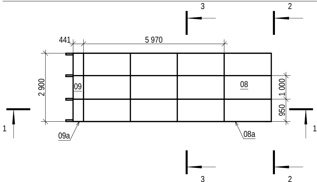
СХЕМА БАЛОК ПАНДУСА 1:100
