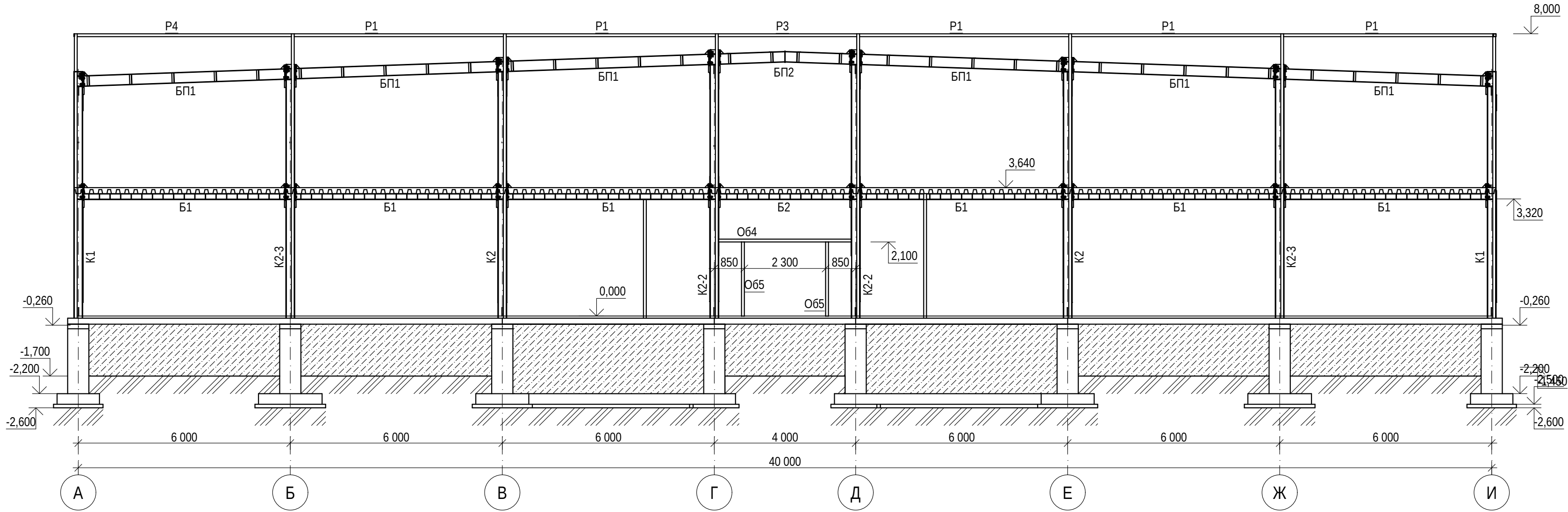
РАЗВЕРТКА И-А/1
