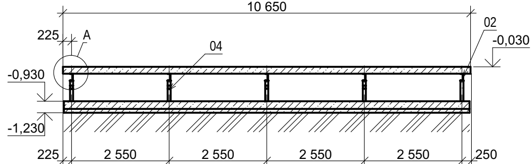
2-2 1:100
