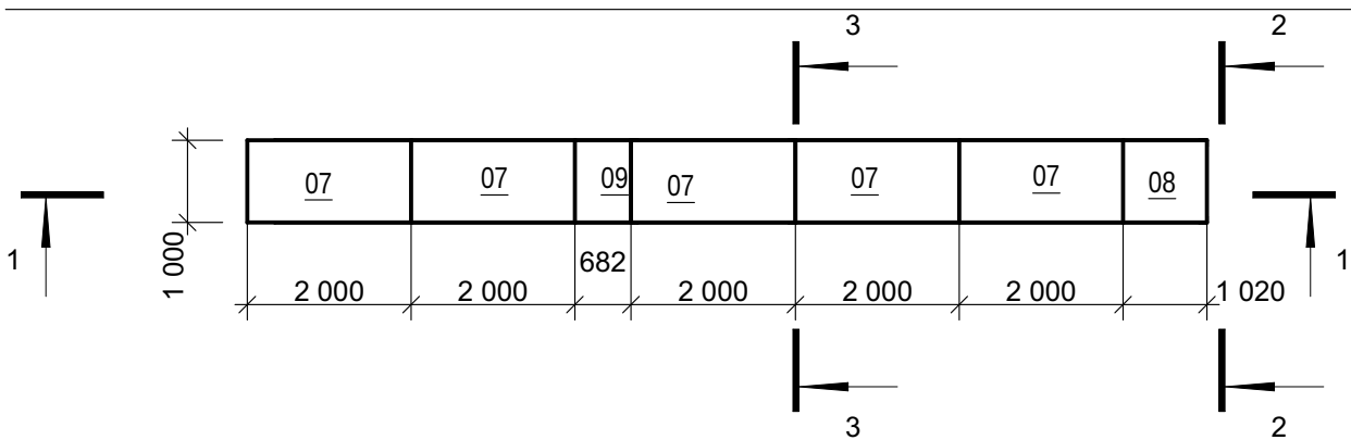
СХЕМА ЛИСТОВ ПОКРЫТИЯ 1:100
